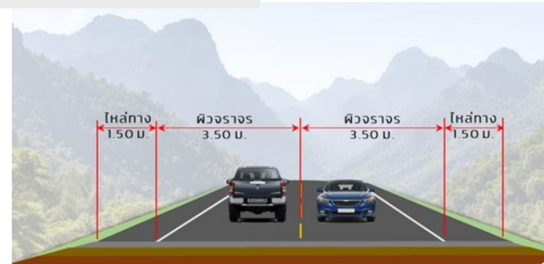
รูปตัดถนนกรณีเขตทางกว้างน้อยกว่า 12 เมตร
